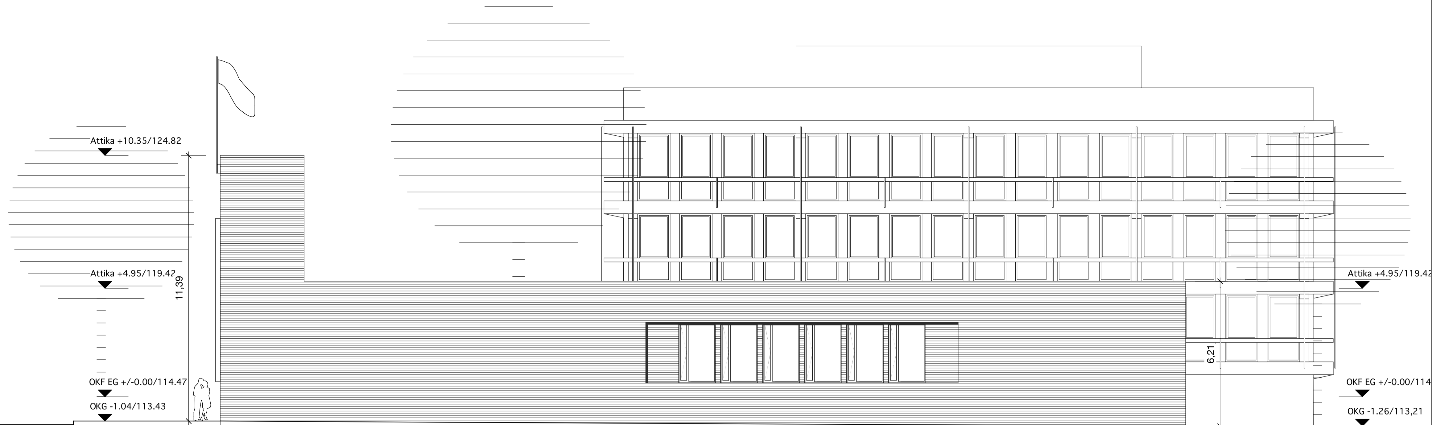
ANSICHT OST M. 1:100
